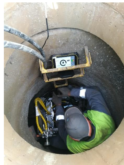
Монтаж оборудования в колодце производится через горловину 60см без демонтажа плиты перекрытия.
